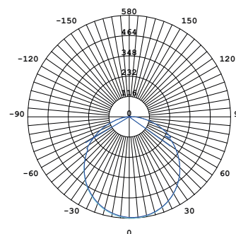
CURVA FOTOMETRICA
